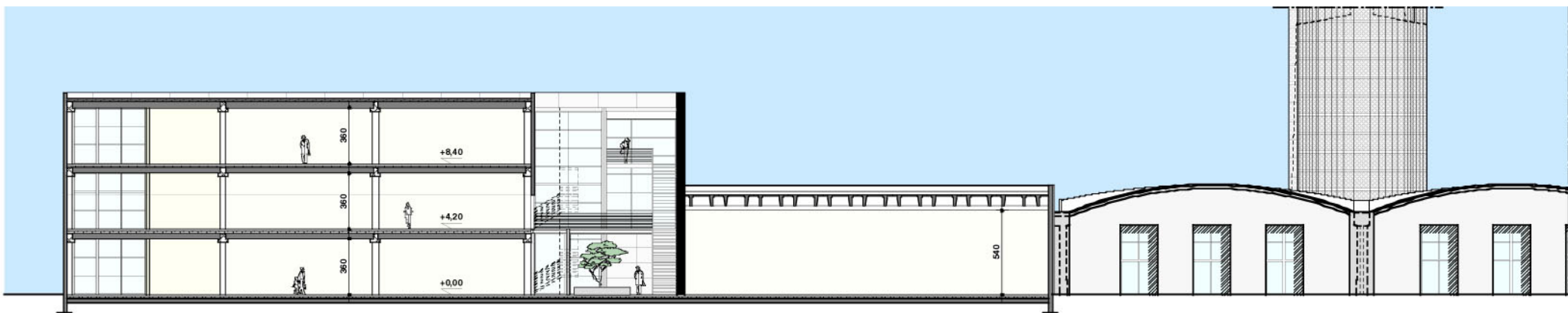
sezione B-B
